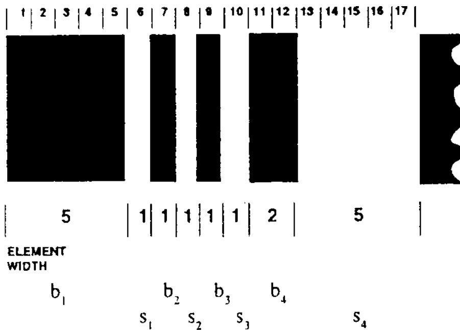
Abbildung 3: Codeword-Symbol
